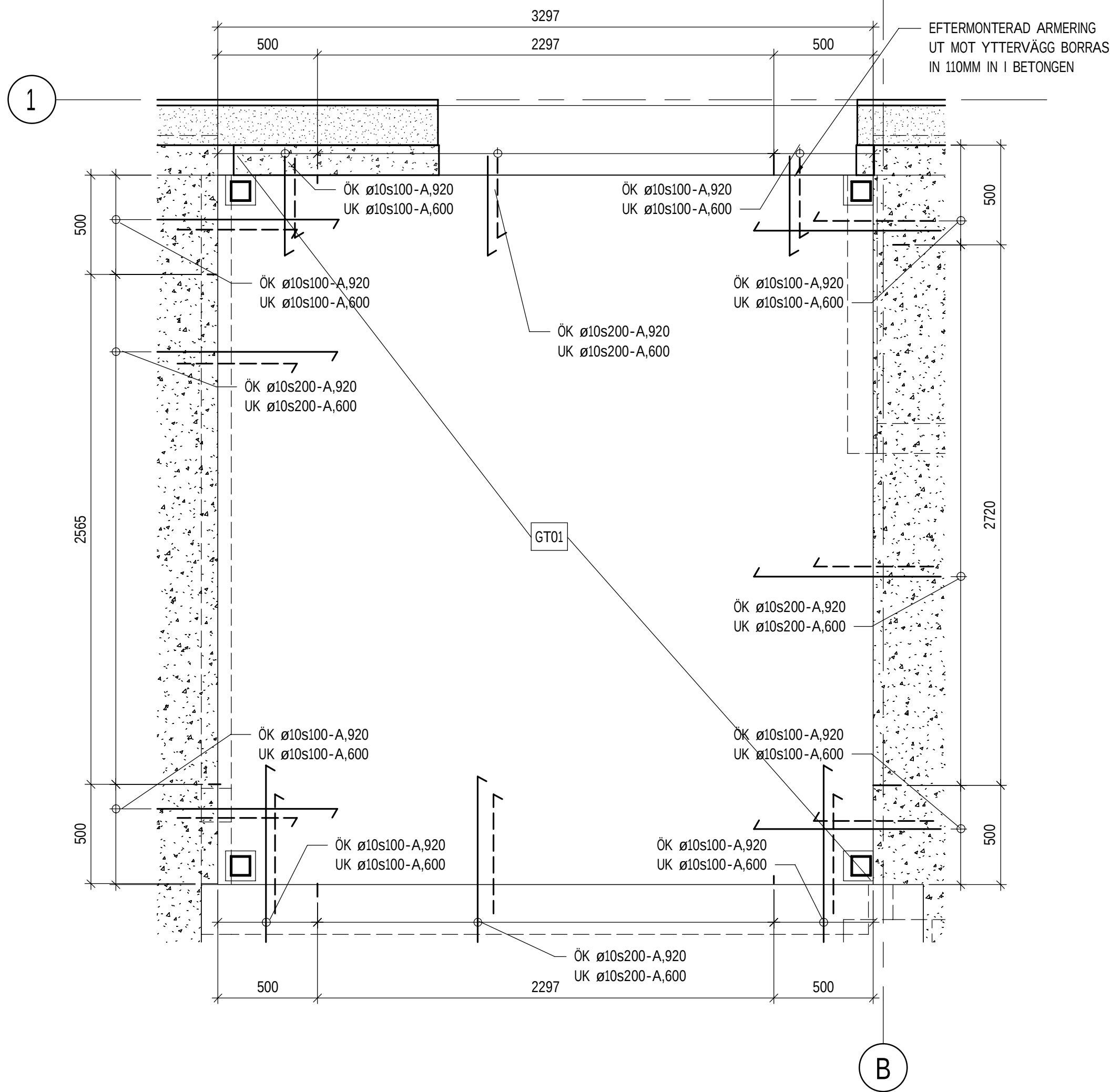
TRAPPHUS PLAN 1 1 : 20
